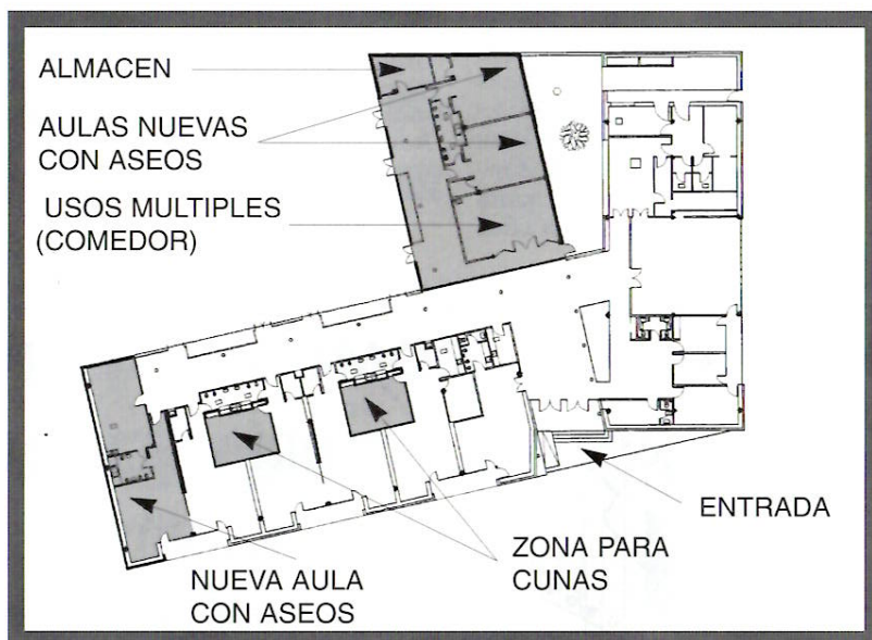
Plano de la Escuela Infantil con detalles de la ampliación y reforma.
